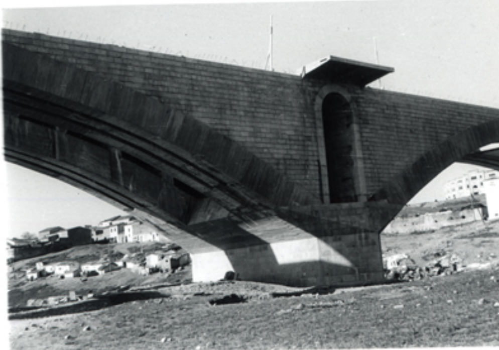
Detalle del puente en construcción
