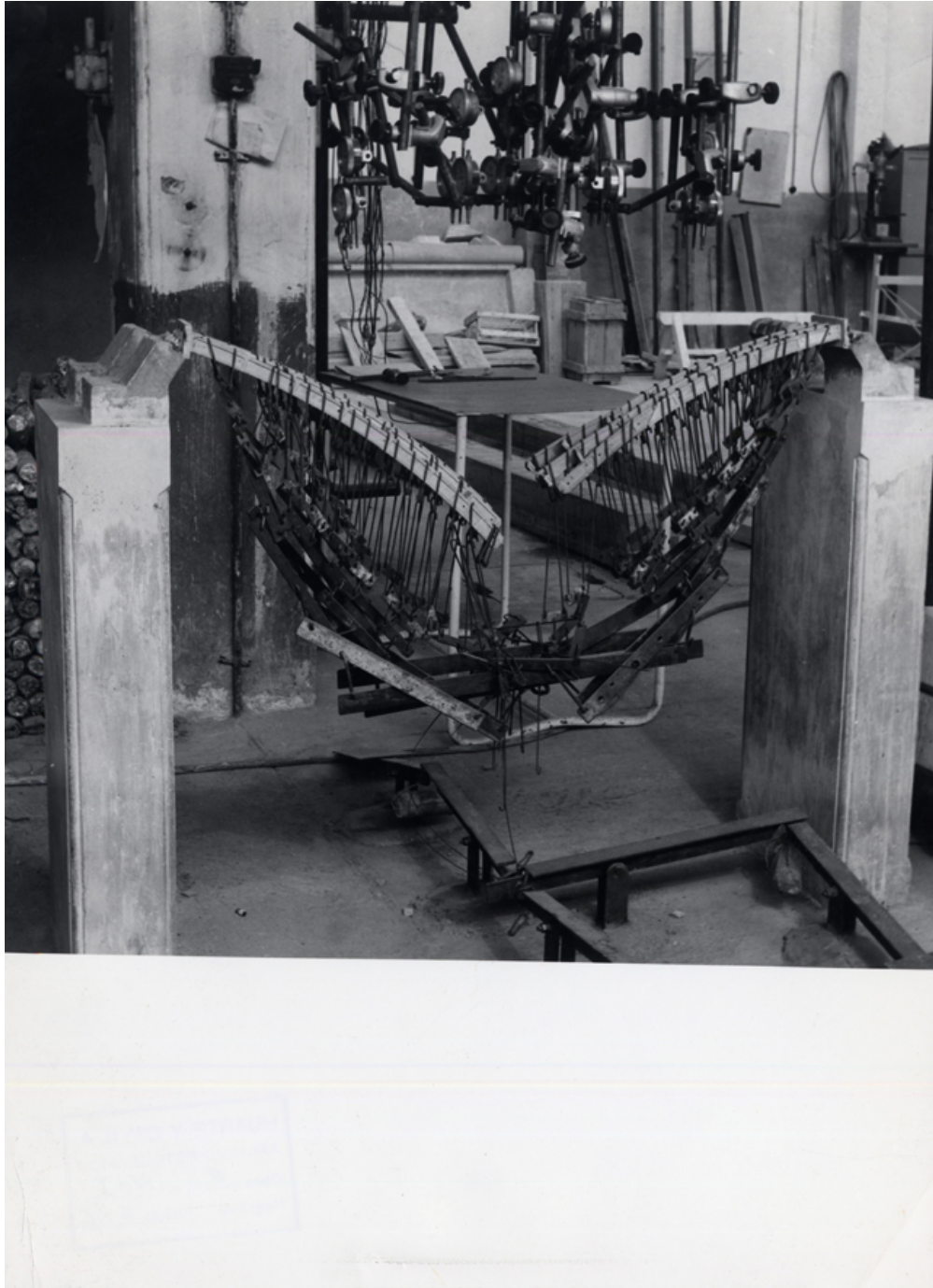
Modelo reducido
