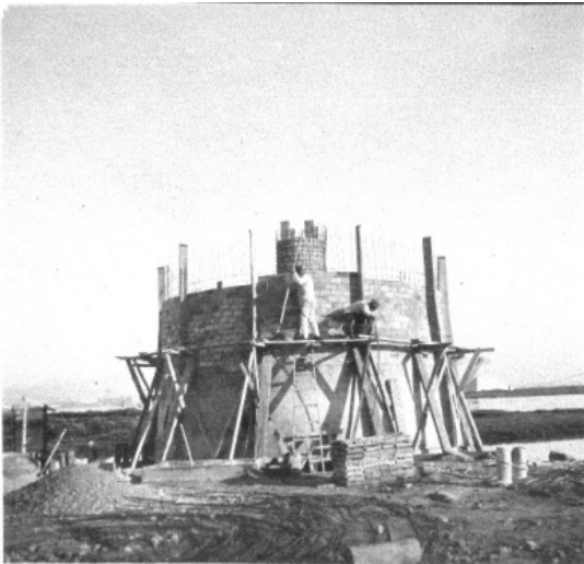
Id: I-ETM-018-03 Título: [Puente de Sancti Petri. Construcción. 2] Fechas: [ca.1927]
