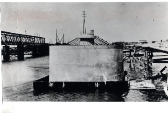
Id: I-ETM-018-06 Título: [Puente de Sancti Petri. Construcción. 5] Fechas: [ca.1927]
