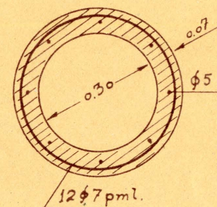
DETALLES DE LA CONDUCCION. ESCALA 1/10
