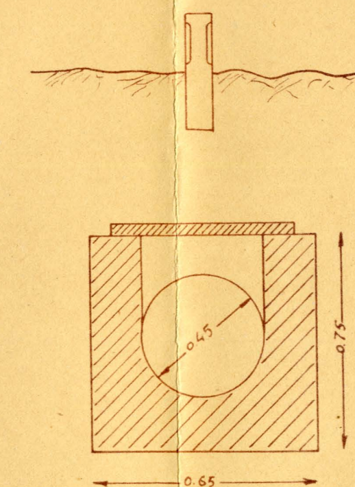
ARQUETA DE REGISTRO ESCALA 1/20
