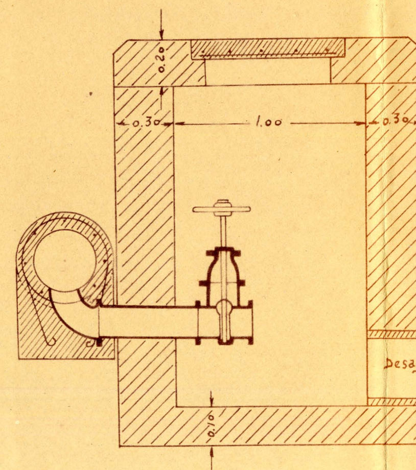
ARQUETA PARA VENTOSA Y DESAGUE DE SIFON. ESCALA 1/20 (Planta Cuadrada)
