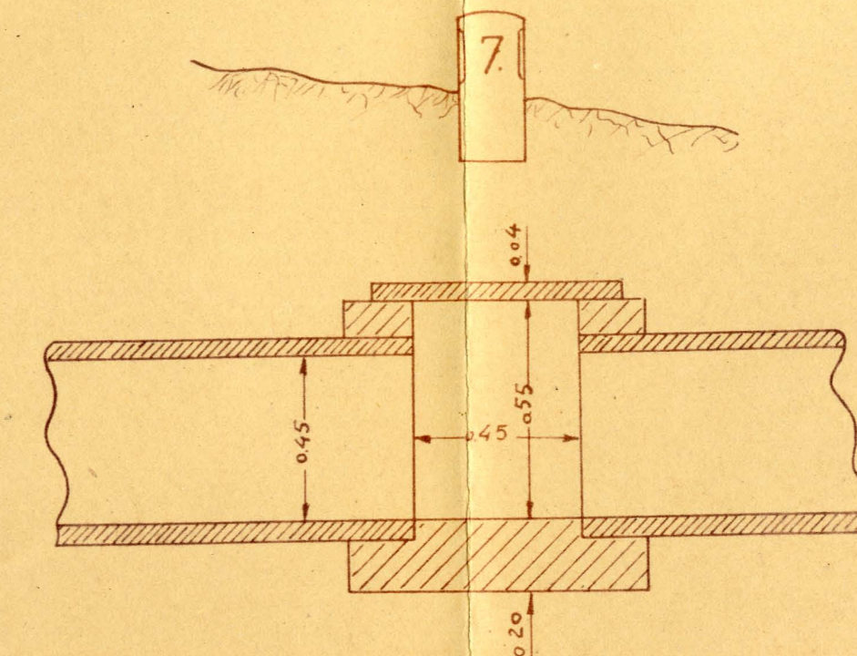
ARQUETA DE REGISTRO ESCALA 1/20
