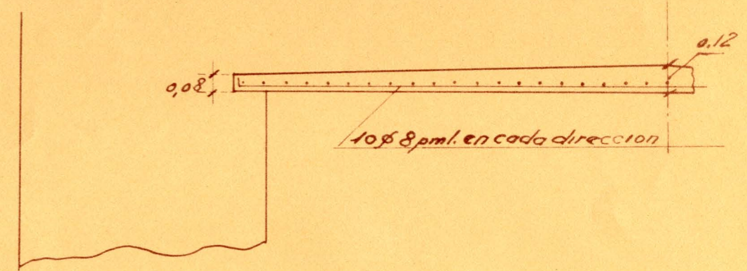
Detalle del forjado de la torre
