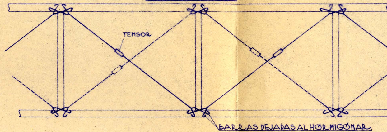
PLANTA DE LOS ARRIOSTRAMIENTOS SUPERIOR E INFERIOR.
