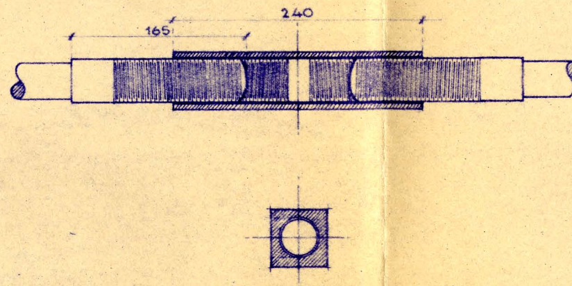
DETALLE DEL TENSOR. Esc. 1:5
