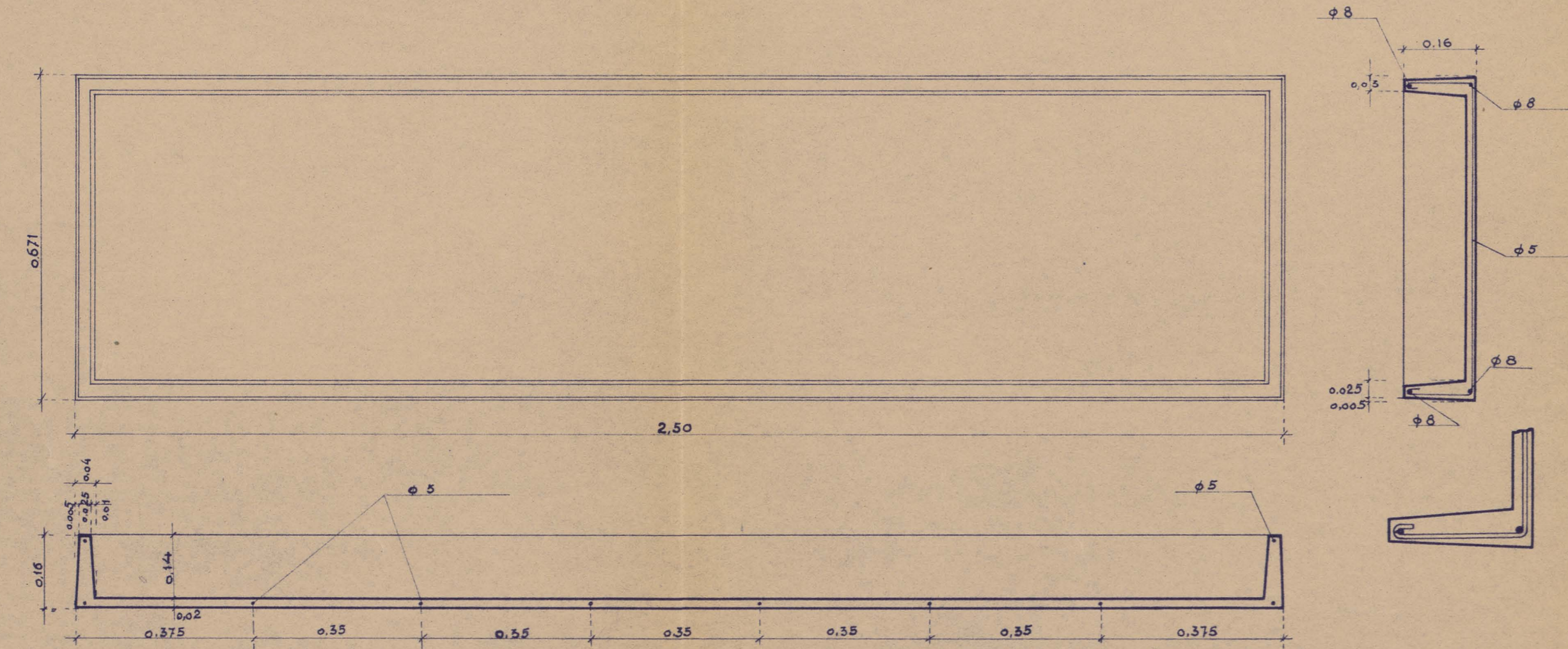
PLACA DE CUBIERTA DE LAS NAVES LATERALES.
