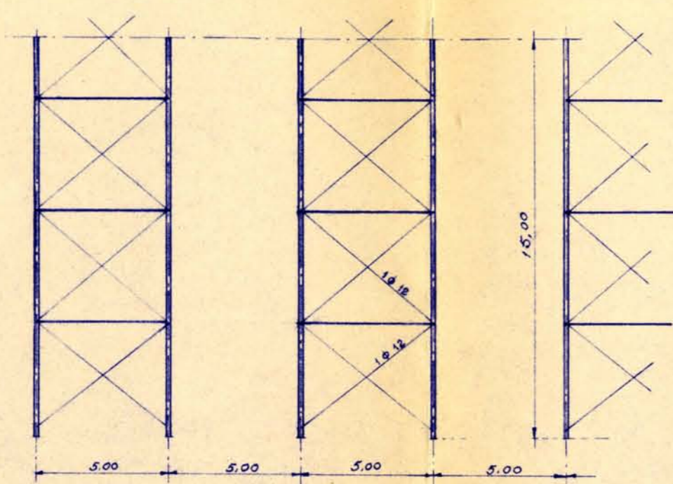
ESQUEMA DEL ARRIOSTRAMIENTO HORIZONTAL
