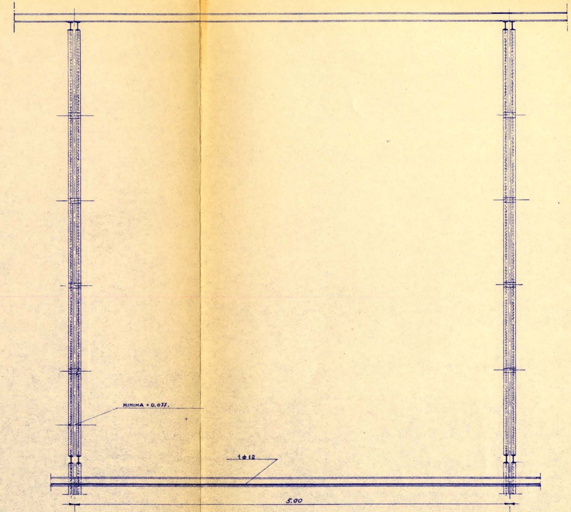
—SECCIÓN 1-1—
