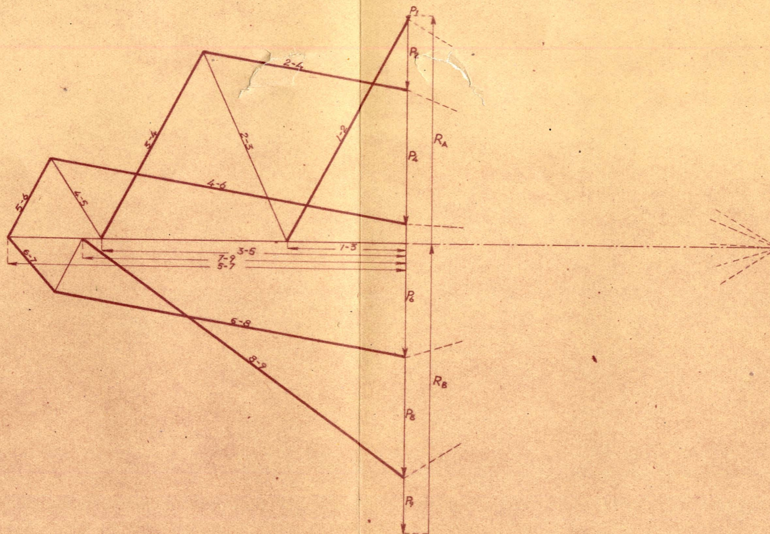
DIAGRAMA DE ESFUERZOS
