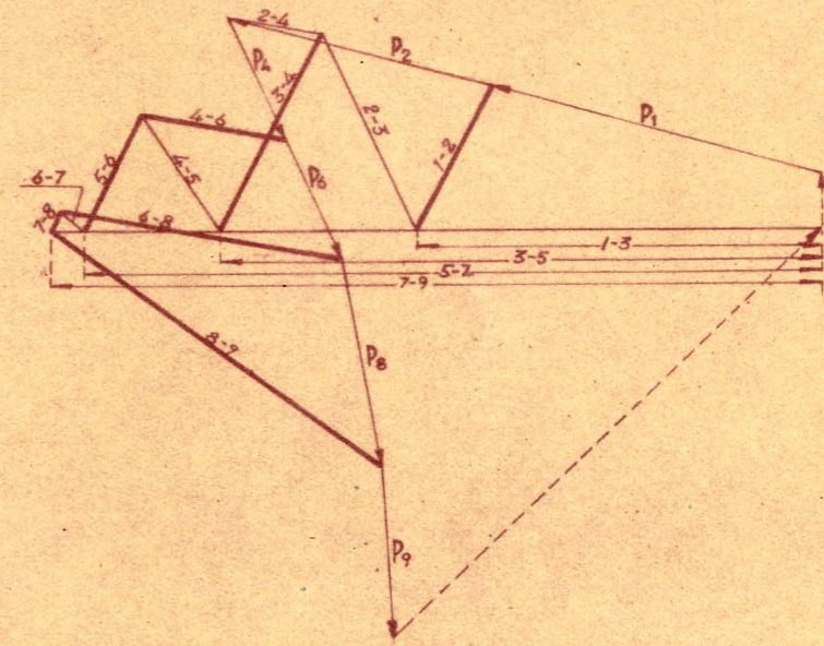
DIAGRAMA DE ESFUERZOS
