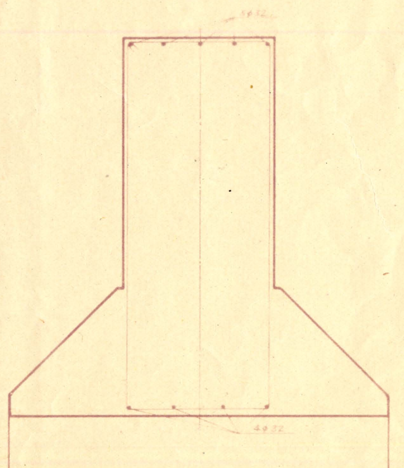
SECCION V-V
