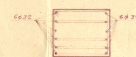
SECCION I-I
