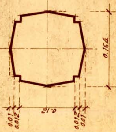
SECCIÓN a-a ESCALA 1:5
